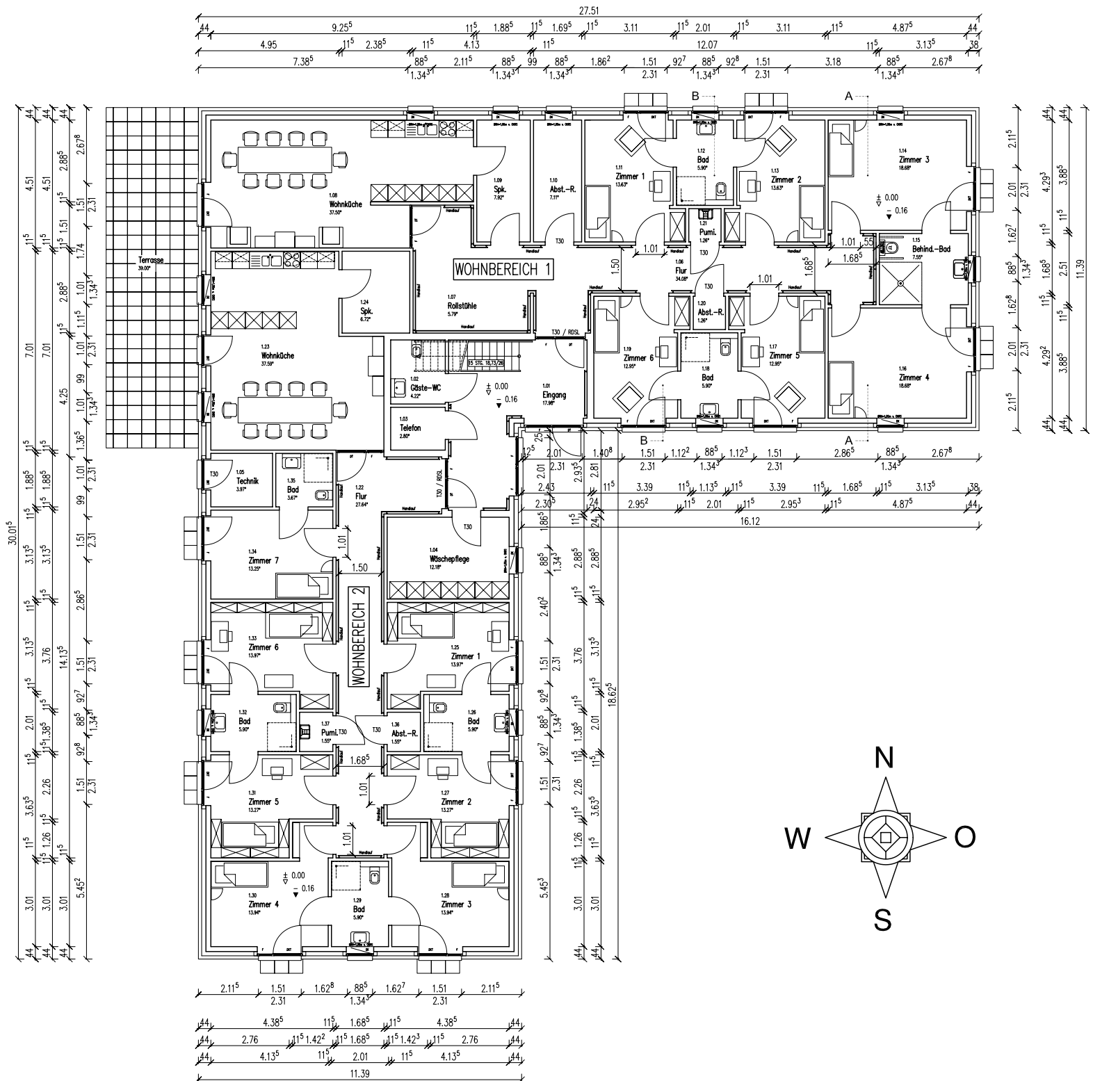
Erdgeschoss
