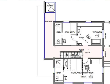
OBERGESCHOSS
