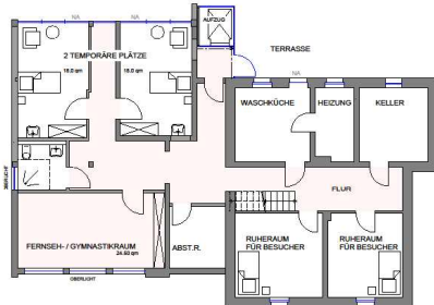
UNTERGESCHOSS
